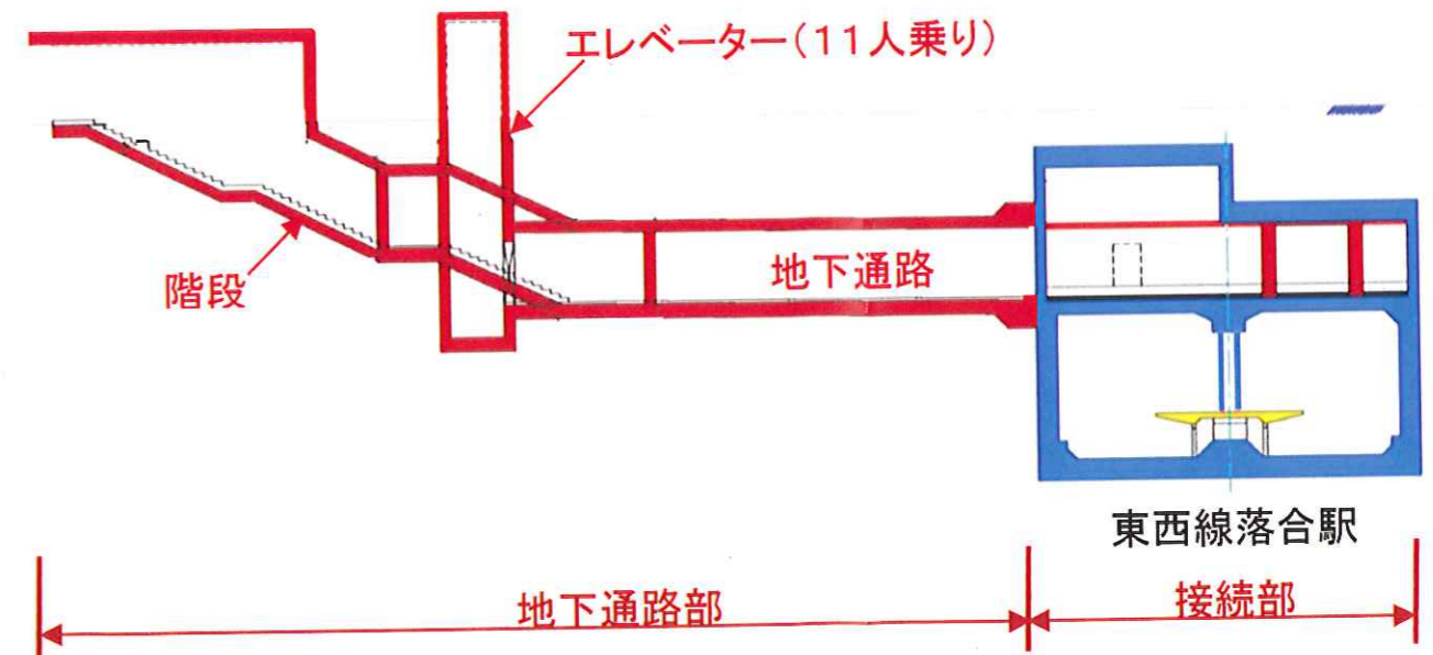
A-A 断面図
